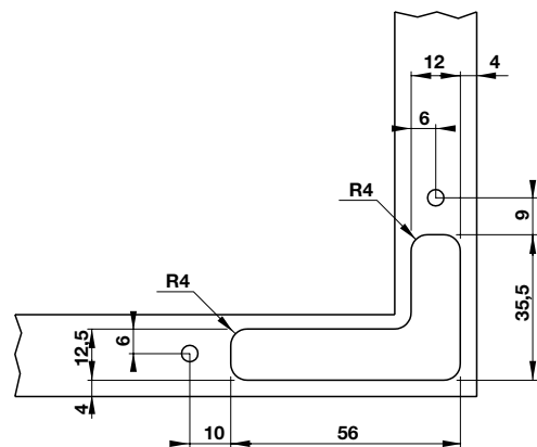
Milling dimension for corner connector Kích thước phay cho bas nối
