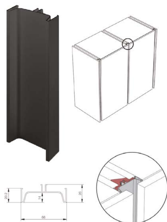
Double / Intermediate Snap-on Vertical Gola Profile Tay nắm dọc đôi Gola/ Lắp giữa
