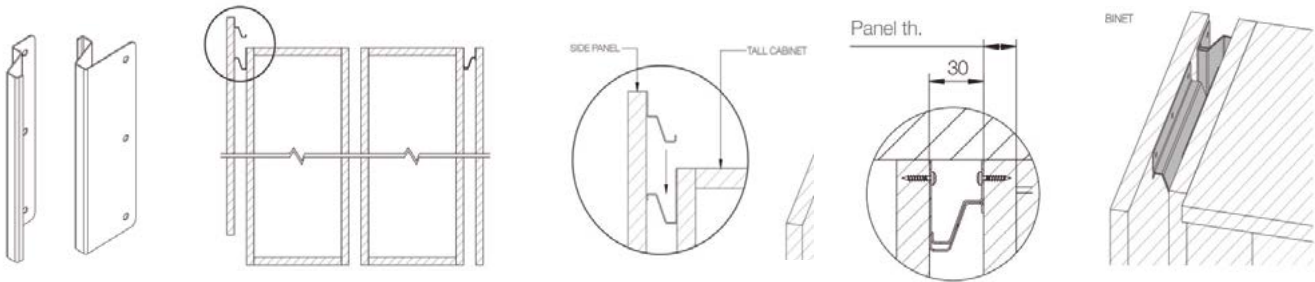
Rear Brackets for Side and Intermediate Snap-on Vertical Gola Profile Bas kết nối rìa cho tay nắm dọc lắp giữa và mặt bên
