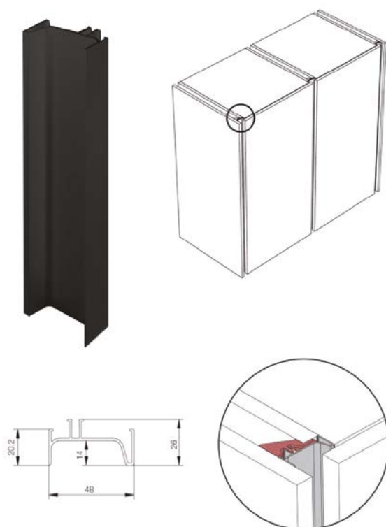
Single / Side Snap-on Vertical Gola Profile Tay nắm dọc đơn Gola/ Lắp mặt bên
