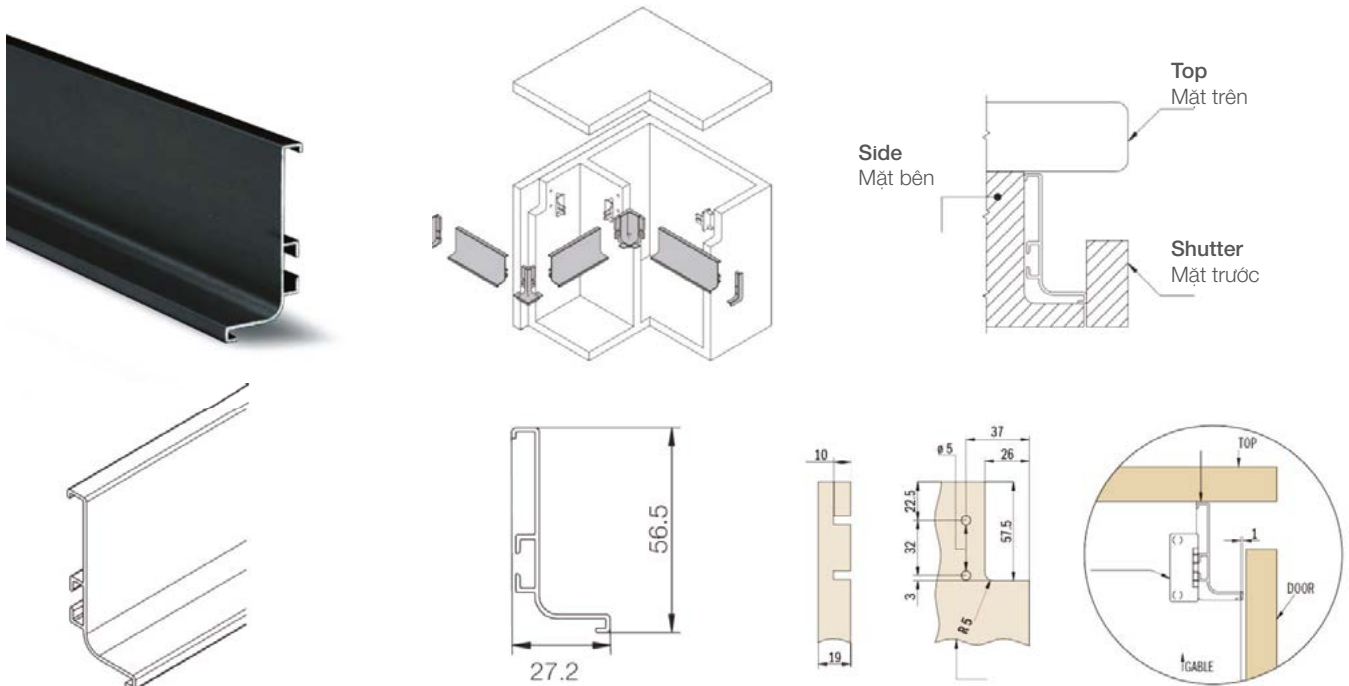
J Gola Profile Tay nắm Gola chữ J
