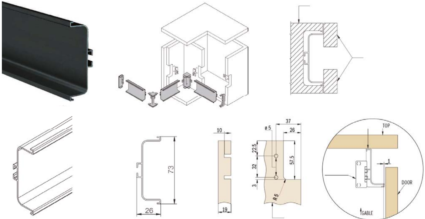
C Gola Profile Side Tay nắm Gola chữ C
