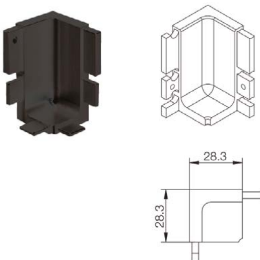
Accessories for J GOLA profile Phụ kiện cho tay nắm GOLA chữ J
