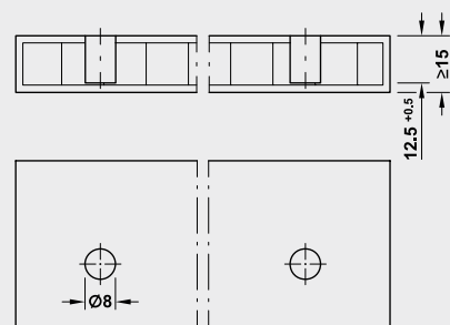
Drill hole on surface / Lỗ khoan trên bề mặt
